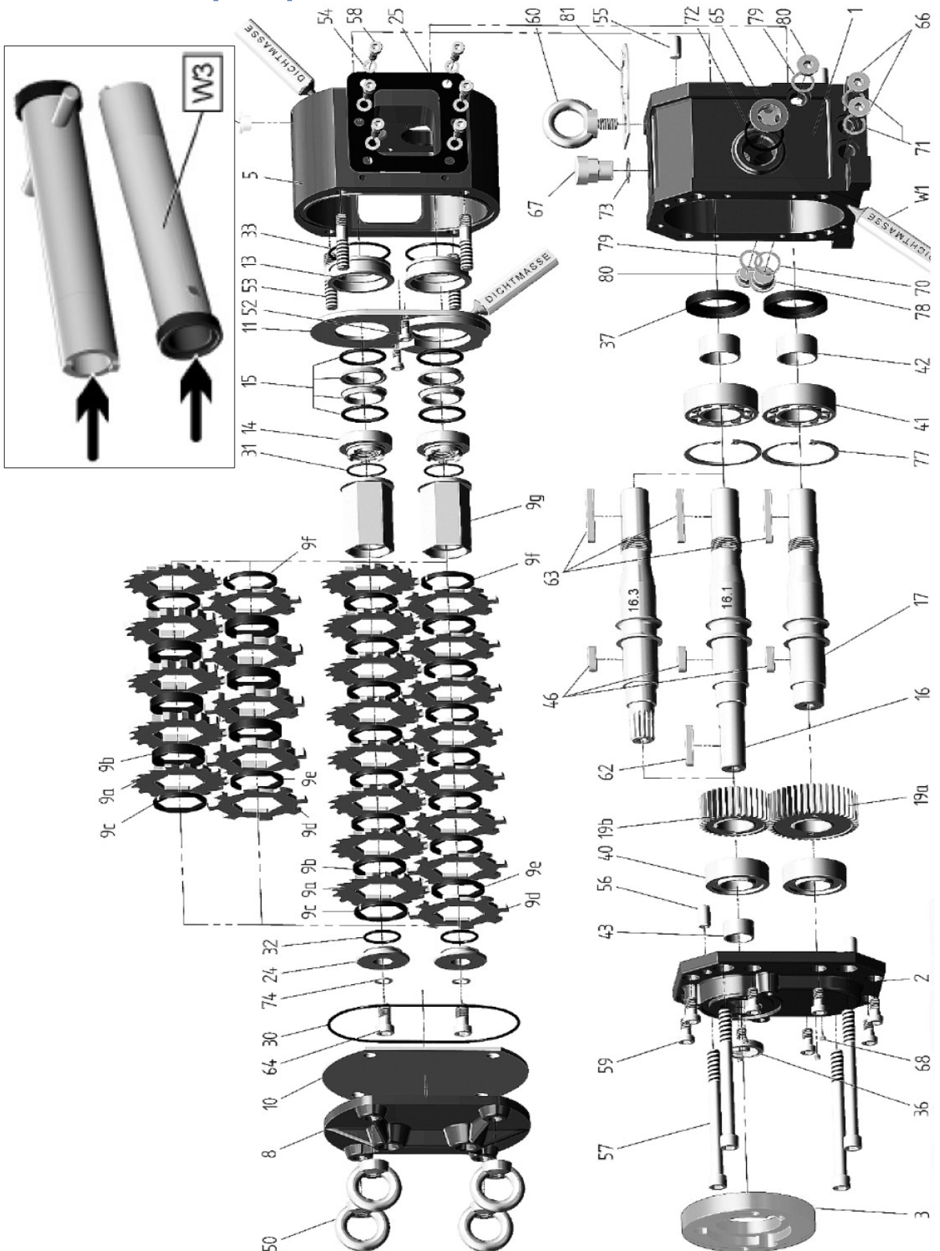
Börger Drehkolbenpumpe Classic Baureihe HAL
