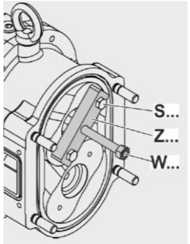
Börger Drehkolbenpumpe Classic Baureihe AN_V1 Detail II
