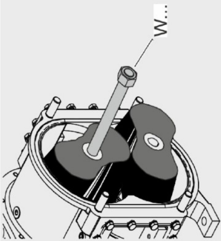
Börger Drehkolbenpumpe Classic Baureihe AN_V1 Detail I
