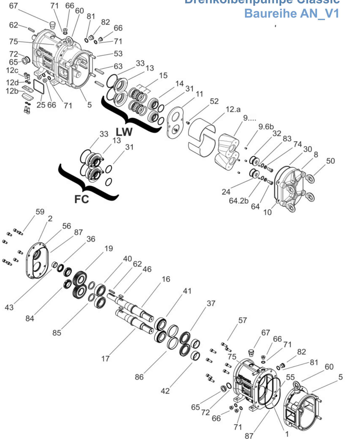
Börger Drehkolbenpumpe Classic Baureihe AN_V1
