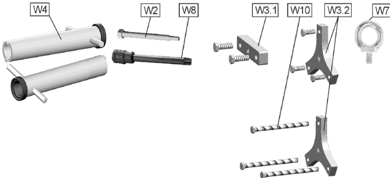
Børgger Drehkolbenpumpe Classic Baureihe EL 1000 und EL 1550 Detail I
