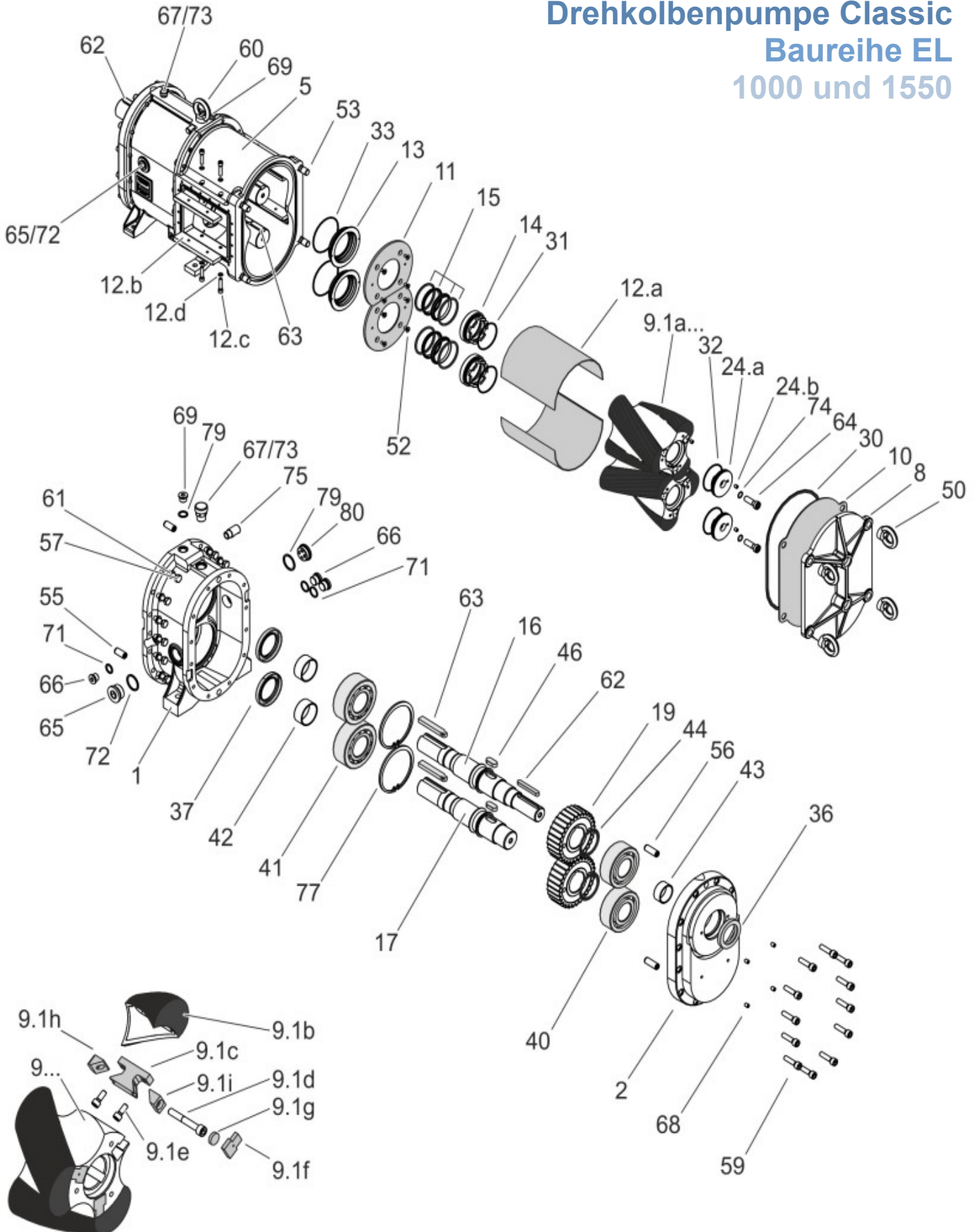
Börger Drehkolbenpumpe Classic Baureihe EL 1000 und EL 1550
