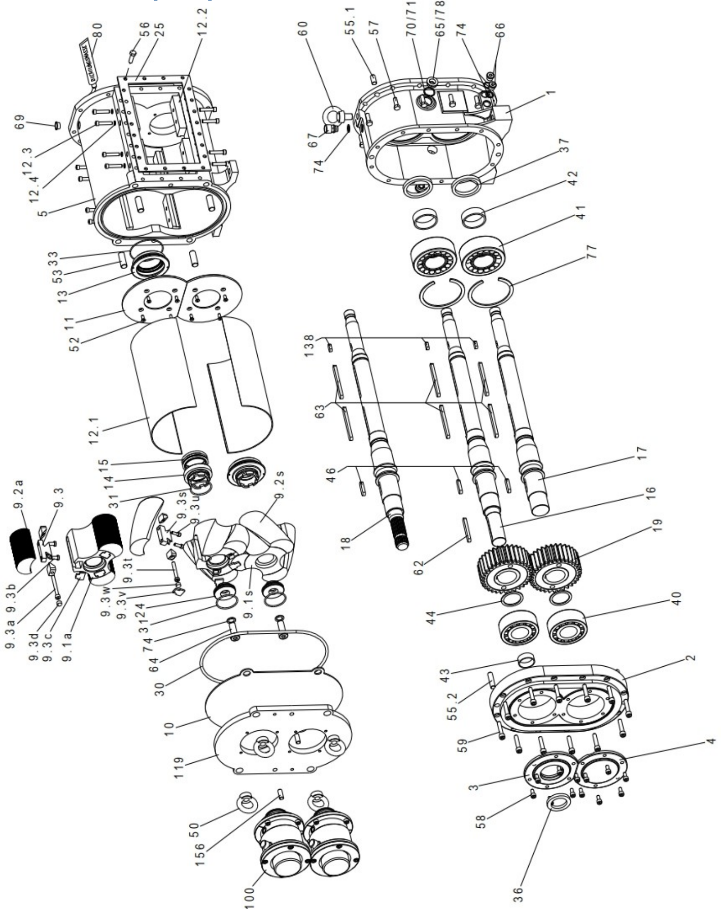
Börger Drehkolbenpumpe Classic Baureihe FLA
