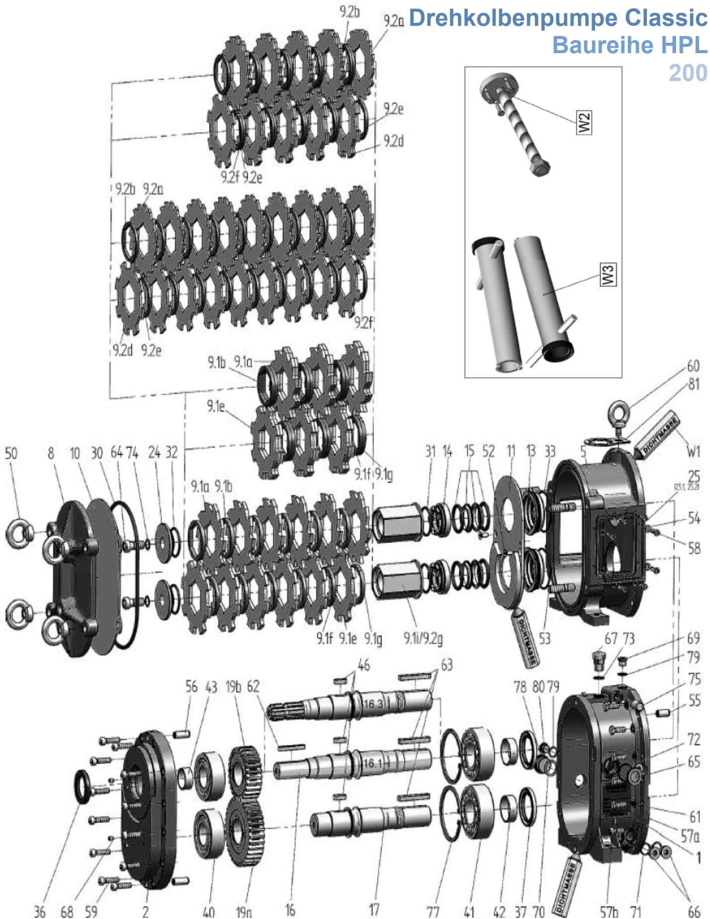
Börger Drehkolbenpumpe Classic Baureihe HPL 200
