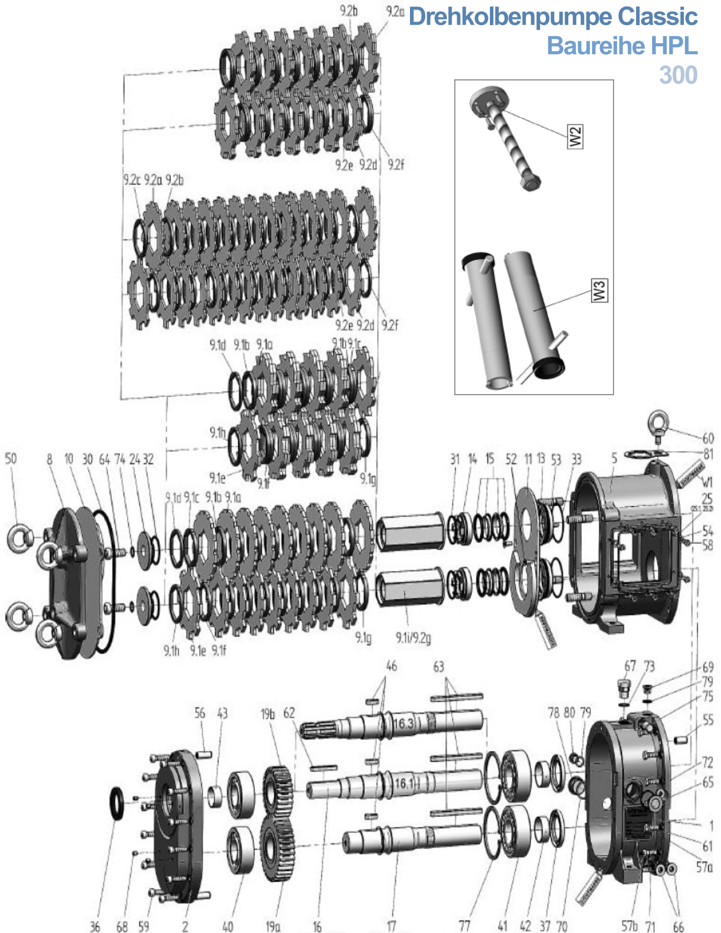
Börger Drehkolbenpumpe Classic Baureihe HPL 300 Seite 1 von 2
